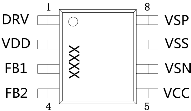
SOP8
