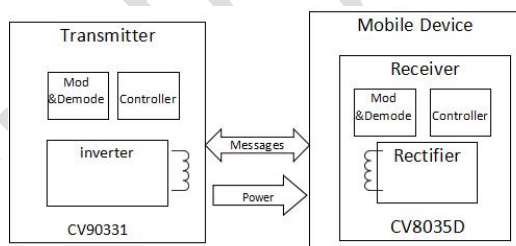
图1. CV90331简化应用电路
